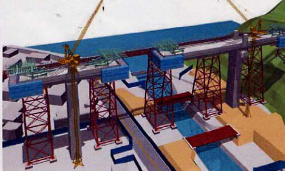
上部工の施工状況（イメージ）
